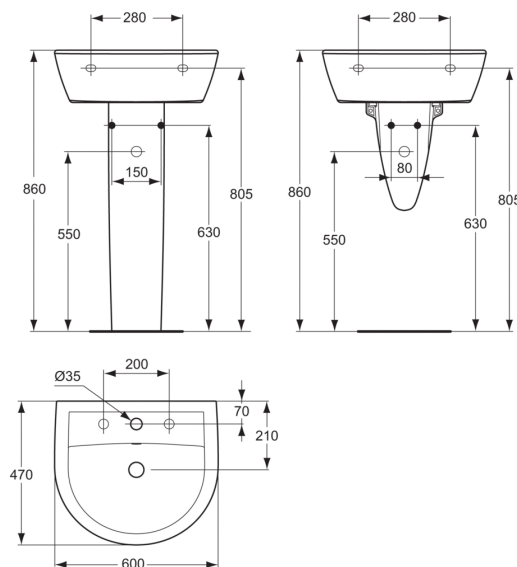
Lavabo mural sur colonne en porcelaine vitrifiée
